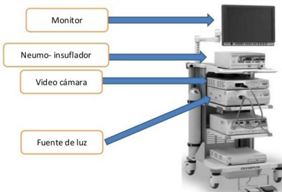
Figura 2. Torre de Laparoscopia
