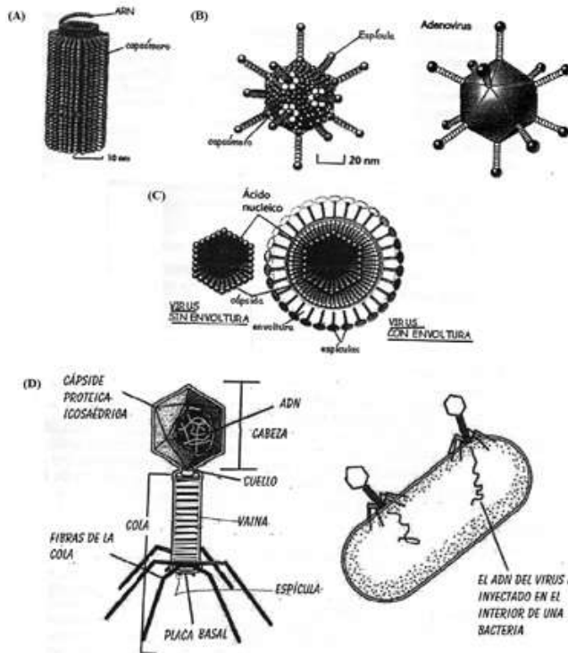
Figura 16. Formas de virus. (A) Virus helicoidal, (B) Virus icosaédrico, (C) Virus sin y con envoltura y (D) Bacteriófago.
