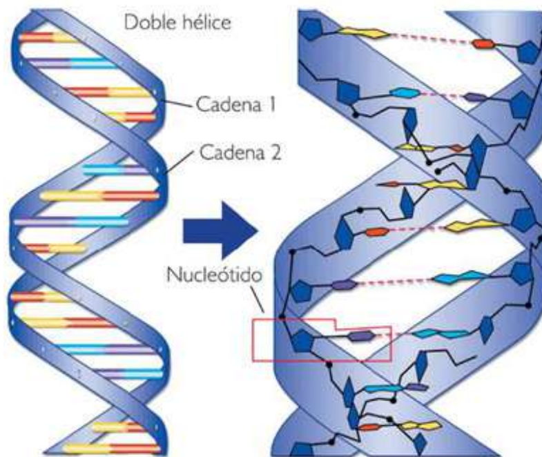
Figura 32. Doble hélice de la estructura de ácidos nucleicos.
