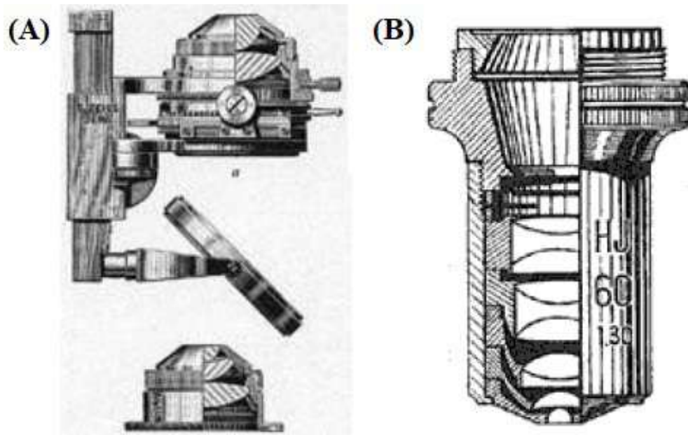
Figura 5. (A) Iluminación del microscopio, fruto de la colaboración de Koch y Abbe y (B) objetivo de inmersión, fruto de la colaboración de Koch y la industria óptica Carl Zeiss.
